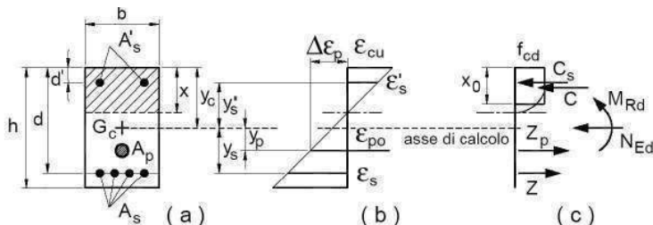
Fig. 4.1.4 – Sezione pressoinflessa
