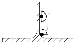
Fig. 4.3.10- Perimetro efficace delle barre di armatura.
