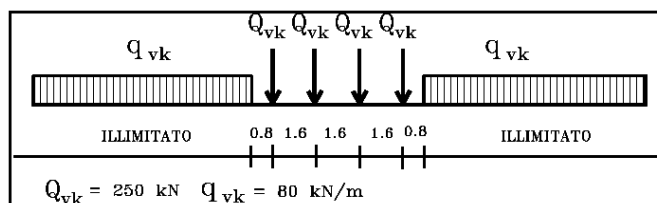
Fig. 5.2.1 - Modello di carico LM71
